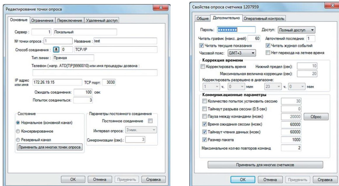
Рисунок 17. Настройки соединения
