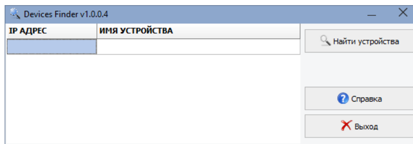
Рисунок 14. Программа “dev_finder”
